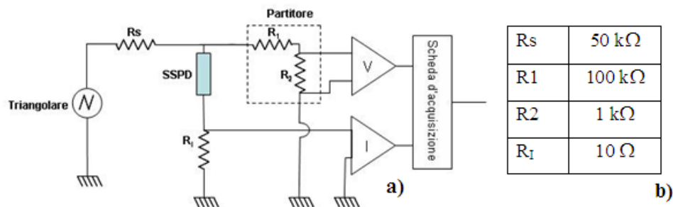
Fig. 76: a) Schema del circuito di acquisizione delle caratteristiche I-V; b) tabella dei valori delle resistenze utilizzate per il circuito di acquisizione
