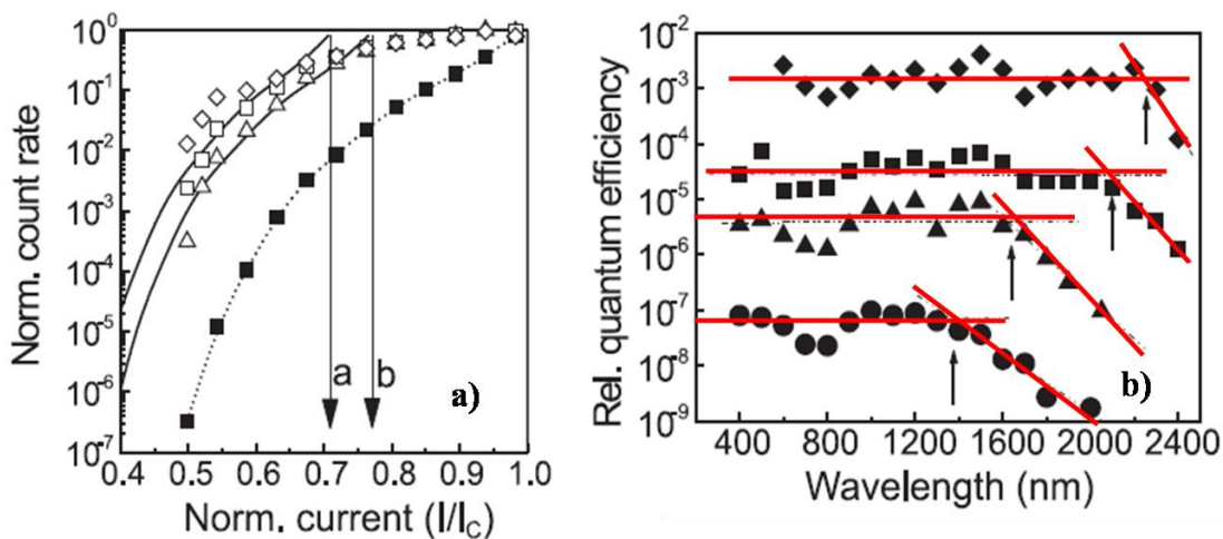
Fig. 7: a) Conteggi al secondo di un SSPD (simboli vuoti) ottenuti a 4.2K per diverse lunghezze d'onda 0,8 \mu m (rombi), 1,2 \mu m (quadrati) e 2 \mu m (triangoli), con i simboli pieni è riportato l'andamento del tasso dei conteggi di buio, tutte le curve sono normalizzate rispetto al loro massimo. b) andamento dell'efficienza quantica relativa misurata per diverse correnti di polarizzazione 0.60 I_c , 0.77 I_c , 0.80 I_c , 0.89 I_c , in funzione della lunghezza d'onda della radiazione incidente, per rendere più facile la lettura del grafico le curve sono state traslate arbitrariamente lungo l'ordinata, le frecce indicano la lunghezza d'onda di soglia [35].
