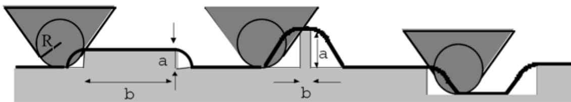
Fig. 45: Effetti di convoluzione tra punta e campione
