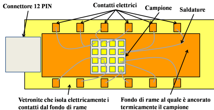
Fig. 48: Porta campioni utilizzato per effettuare la caratterizzazione elettrica a 4.2K dei dispositivi.
