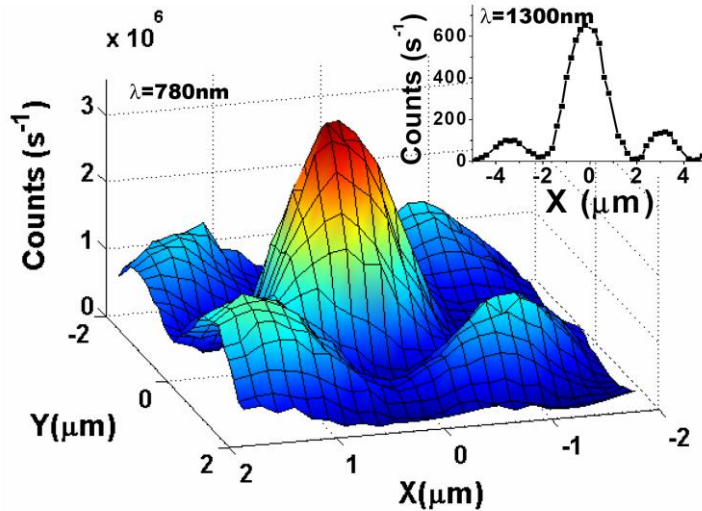
Fig. 91: Immagine in due dimensioni dei conteggi del rivelatore in funzione della posizione dello spot del laser ( \lambda=780\text{nm} , numero di fotoni \gg 1 ). Nell'inserto una scansione in una dimensione ( \lambda=1300\text{nm} e 0.5 fotoni in media per impulso).
