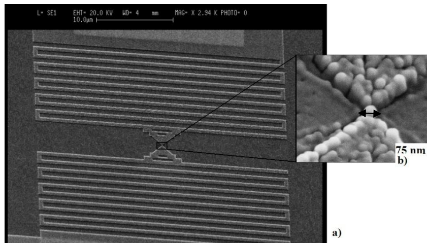
Fig. 74: a) Immagine a scansione elettronica di un SPC largo 75nm, a nord e a sud del dispositivo è possibile vedere l'induttore di NbN inserito per rallentare il dispositivo ed impedire la formazione di uno stato resistivo stabile; b) ingrandimento del punto di contatto di 75nm.
