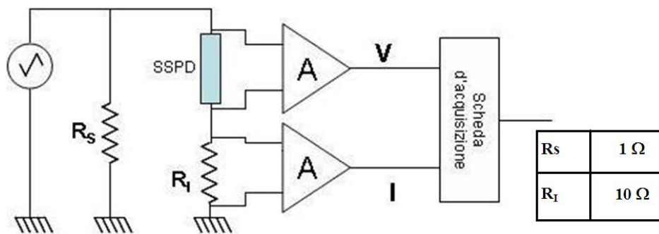
Fig. 78: Schema del circuito utilizzato per l'acquisizione delle caratteristiche IV del hotspot plateau ;
