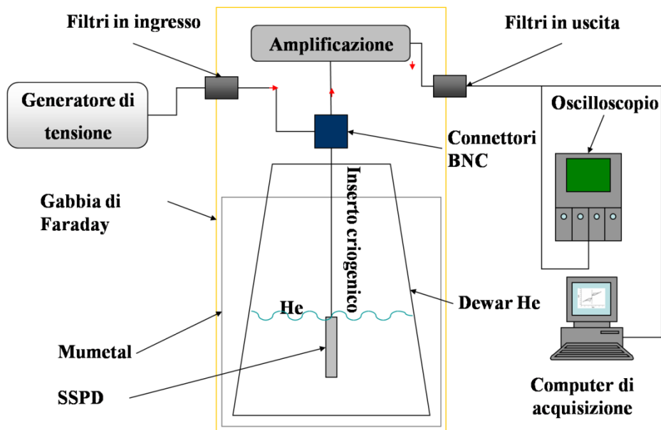
Fig. 49: Schema di principio dell'apparato sperimentale utilizzato per l'acquisizione a 4.2K delle caratteristiche IV.
