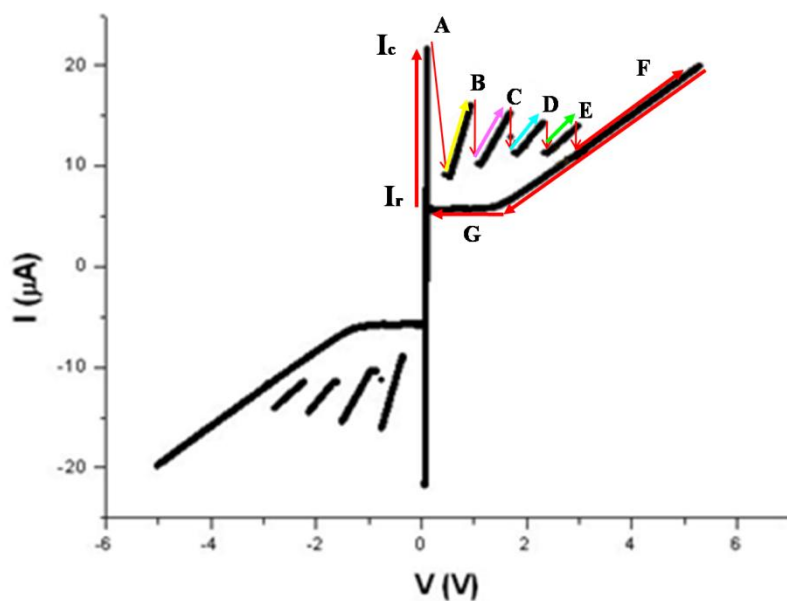
Fig. 77: Caratteristica IV di un meandro costituito da 5 fili in serie. Le lettere indicano l'ordine con cui, aumentando la corrente di polarizzazione I_b oltre il valore della corrente critica I_c , transiscono i 5 fili (da A fino ad E), mentre seguendo le frecce si ha un'idea di come si sviluppa la caratteristica IV.
