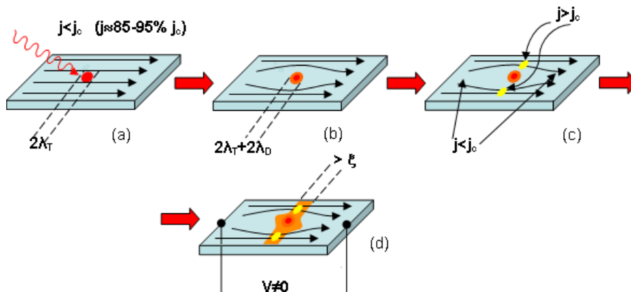
Fig. 2: Schema del meccanismo di rivelazione di un singolo fotone in un SSPD.
