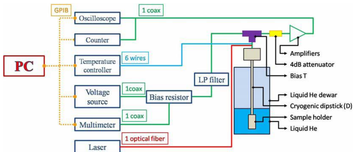
Fig. 52: Diagramma a blocchi dell'apparato utilizzato per la caratterizzazione degli SSPD a 4.2K. il controllo della temperatura è eseguito con un Lake Shore 325, il generatore di tensione continua è un Yokogawa 7651, il multimetro un HP3458A, il contatore uno Standford research system SR 400, l'oscilloscopio un Tektronix TDS 5104 (1 GHz bandwidth) o un Agilent Infiniium DCA-J 86100 C (40 GHz bandwidth)
