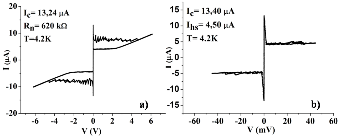
Fig. 80: a) Caratteristica IV ottenute a 4.2K con un meandro costituito da un nanofilo di NbN su MgO largo 100nm, lungo 105 \mu m e spesso 5nm; b) caratteristica IV del hotspot plateau ottenuta con lo stesso dispositivo sempre a 4.2K
