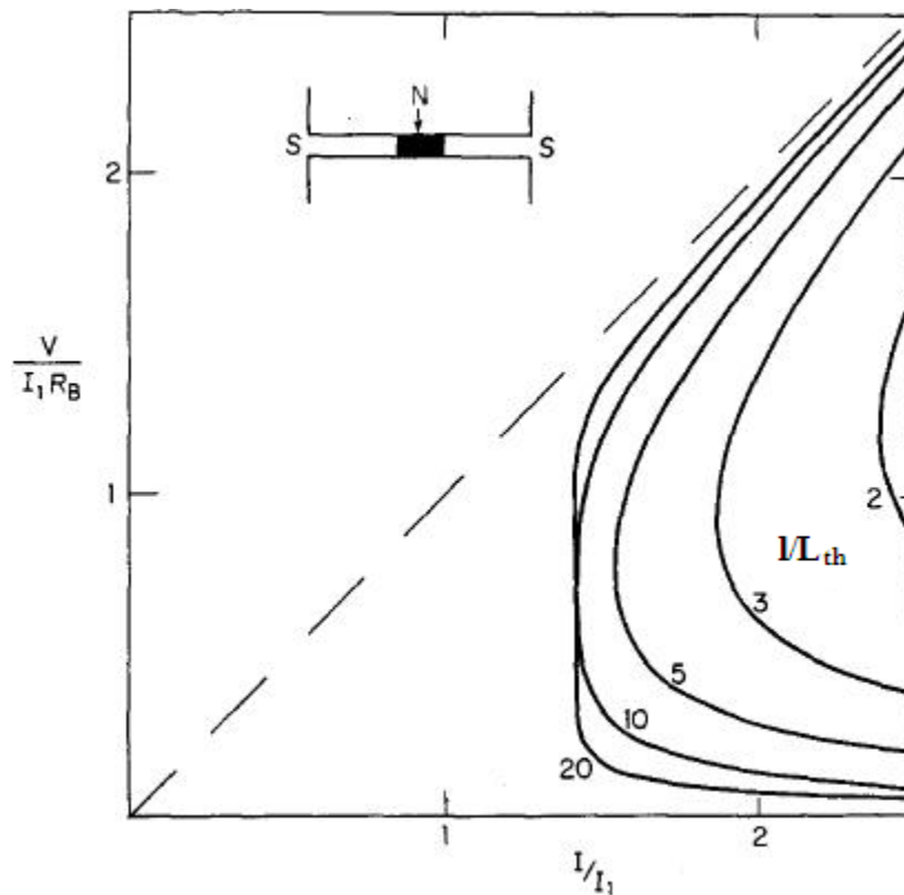
Fig. 20: Andamento teorico delle caratteristiche IV ottenuto tramite il modello di SBT. I_1 e R_B sono definite nel testo. Nel riquadro viene riportata la geometria utilizzata per derivare il modello. I numeri riportati affianco ad ogni caratteristica indicano il corrisponde valore del rapporto l/L_{th} tra la lunghezza del nanofilo l e quella di termalizzazione L_{th} .
