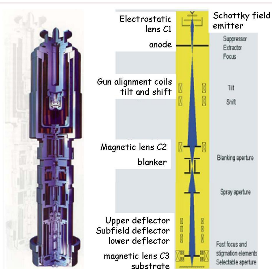
Fig. 27: Schema della colonna elettro-ottica dell'apparato litografico EBPG 5 HR
