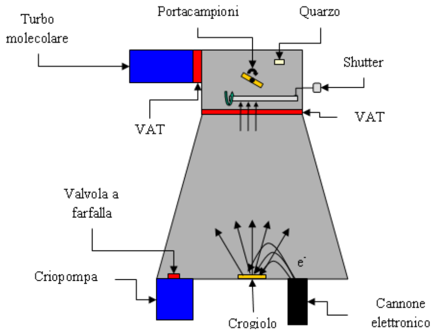
Fig. 30: Schema di funzionamento dell'evaporatore a cannone elettronico. Gli elettroni emessi da un filamento ed accelerati vanno a colpire un crogiolo con il materiale da evaporare. Il vapore così prodotto va a condensare sulle pareti della camera e sul campione
