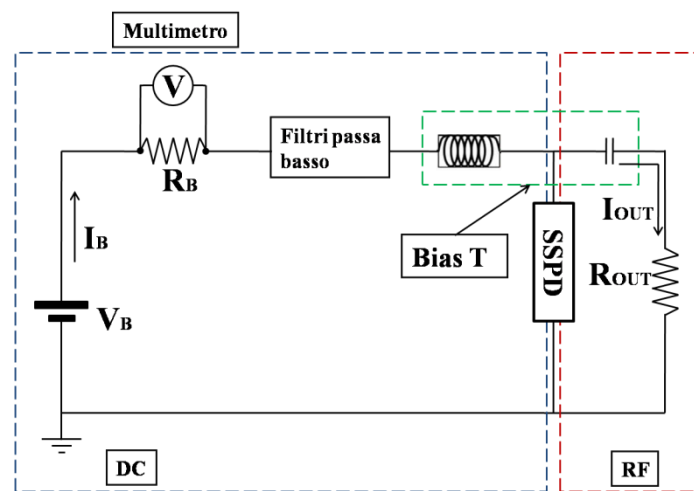
Fig. 82: Circuito equivalente dell'apparato utilizzato per la caratterizzazione ottica
