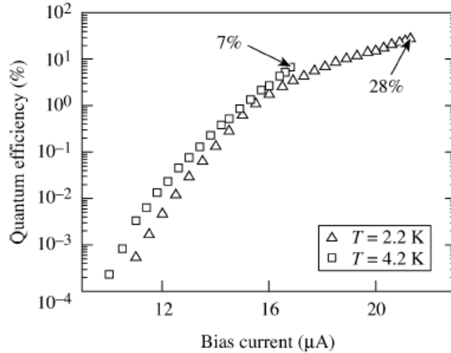
Fig. 9: Andamento dell'efficienza quantica per due temperature di lavoro diverse (2.2K e 4.2K) e \lambda=1.26 \mu\text{m} . Come è possibile notare la QE aumenta con il diminuire della temperatura [28].
