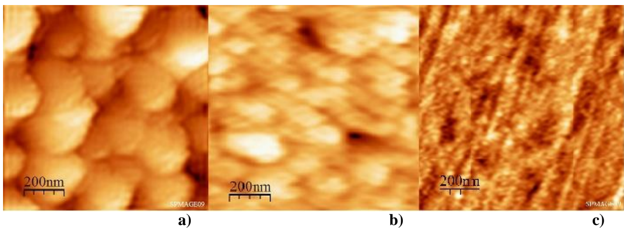
Fig. 62: Immagini AFM delle superfici dei tre campioni riscaldati a tre temperature diverse per 8 ore, a) 400°C, b) 350°C e c) a 300°C.
