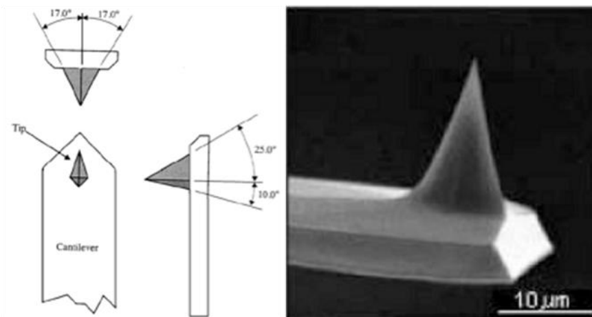
Fig. 44: Angoli tipici d'inclinazione delle pareti laterali di una sonda di silicio
