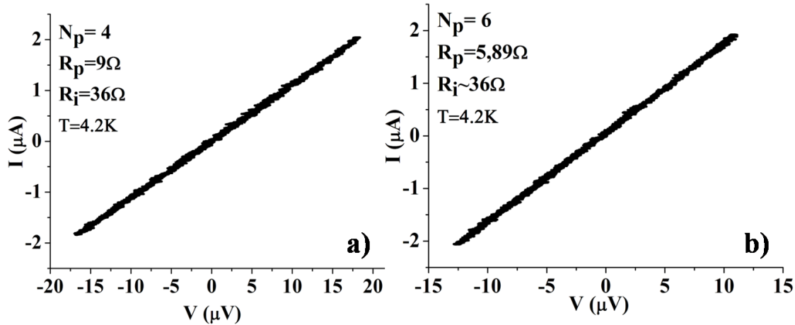
Fig. 95: Misura a 4.2K del valore della resistenza risultante dal parallelo delle resistenze serie dei diversi elementi del PND. In questo caso la misura è stata effettuata a quattro fili in modo da eliminare la resistenza di circa 20 \Omega dovuta ai fili con i quali il dispositivo è collegato con gli strumenti all'esterno del dewar.
