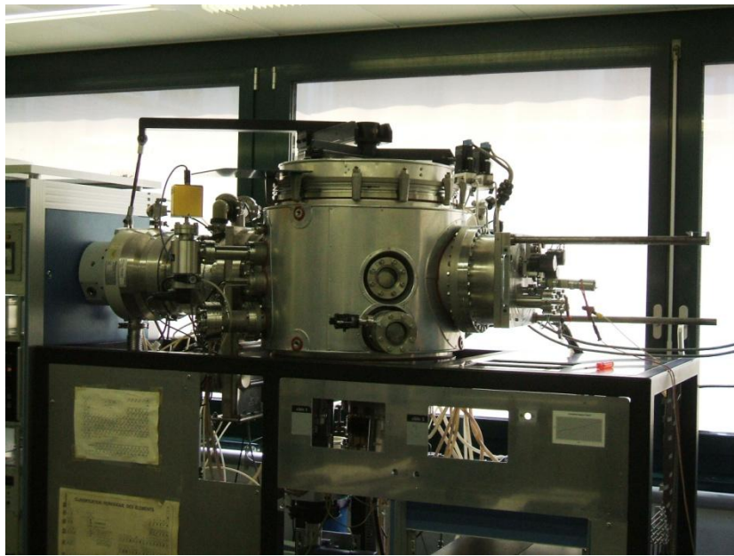
Fig. 32: Impianto per la crescita tramite sputtering utilizzato per la deposizione dei film superconduttori.
