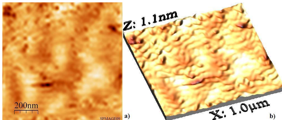
Fig. 64: a) Immagine AFM 2D della superficie di un film di NbN deposto su GaAs dopo l'ottimizzazione del processo, l'area di scansione è di 1\mu\text{m}^2 , b) la stessa immagine in 3D.
