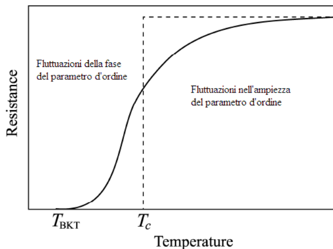
Fig. 10: Transizione resistiva in un superconduttore 2D. Al di sopra di T_c la transizione è dominata dalle fluttuazioni dell'ampiezza del parametro d'ordine, mentre al di sotto da quelle della fase del parametro d'ordine, finché non si arriva a T=T_{BKT} , quando finalmente R diventa zero.
