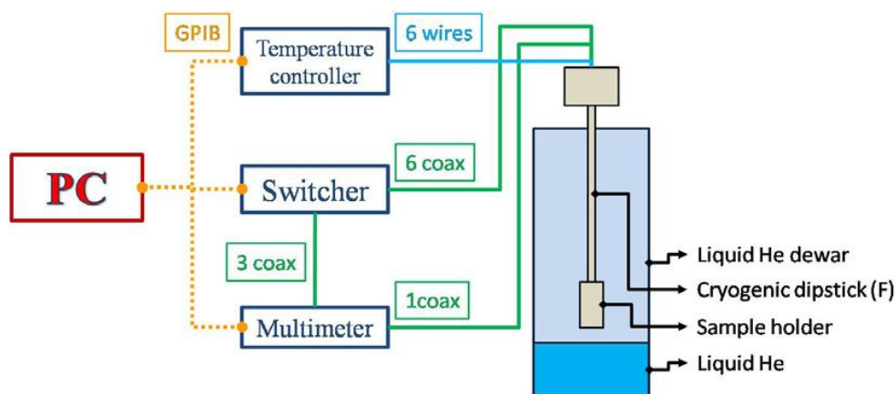
Fig. 46: Diagramma a blocchi dell'apparato utilizzato per le misure della resistenza in funzione della temperatura. Il controllo della temperatura viene eseguito tramite un Conductus LTC10 o un Lake Shore 325, lo switcher è un HP 3488A, mentre il multimetro un HP 3458A.
