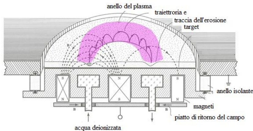
Fig. 31: Sezione trasversale della struttura del magnete planare circolare. Il raggio delle orbite degli elettroni non è in scala per una migliore comprensione, [84].
