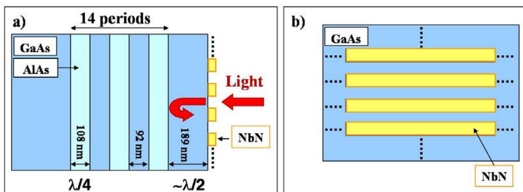
Fig. 54: a) Visione laterale e b) frontale della struttura del DBR utilizzata per le simulazioni dei DBR
