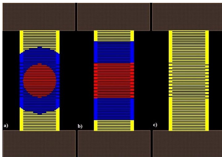
Fig. 71: Esempi di simmetrie di dose utilizzate per la correzione dell'effetto di prossimità su GaAs, a) simmetria circolare, b) simmetria quadrata, ogni colore corrisponde ad una dose diversa, più alta all'esterno (giallo) e minore al centro (rosso); c) simmetria utilizzata per la realizzazione di un meandro su MgO dove non è necessaria alcuna correzione dell'effetto di prossimità
