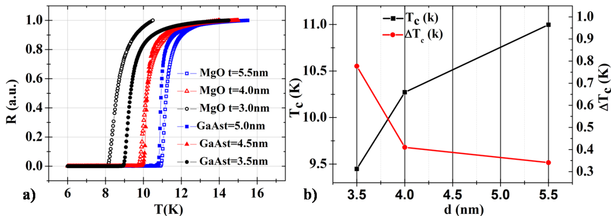
Fig. 65: a) Confronto tra l'andamento della resistenza in funzione della temperatura dei film di NbN deposti su GaAs in seguito al processo di ottimizzazione (simboli chiusi) e dei film deposti su MgO. Il colore identifica spessori confrontabili entro l'errore della misura ( \pm 0.5\text{nm} ); b) andamento della temperatura critica T_c e della larghezza di transizione \Delta T_c in funzione dello spessore.
