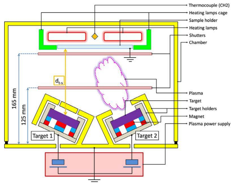
Fig. 33: Schema illustrativo della camera di deposizione dell'impianto da sputtering utilizzato per la crescita dei film di NbN
