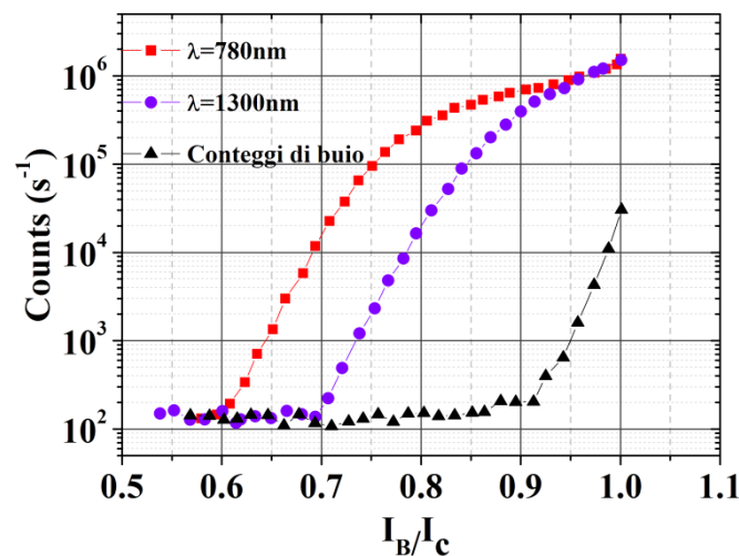
Fig. 87: Risposta ottica di un SSPD costituito da un nanofilo largo 100nm lungo 105 \mu\text{m} avvolto a meandro con un fattore di riempimento pari al 40%, con i quadrati rossi è rappresentata la risposta del rivelatore ad una radiazione incidente di lunghezza d'onda pari a \lambda=780\text{nm} , con i cerchi viola quella del rivelatore ad una radiazione di lunghezza d'onda pari a 1.3 \mu\text{m} , mentre con i triangoli neri sono indicati i conteggi di buio
