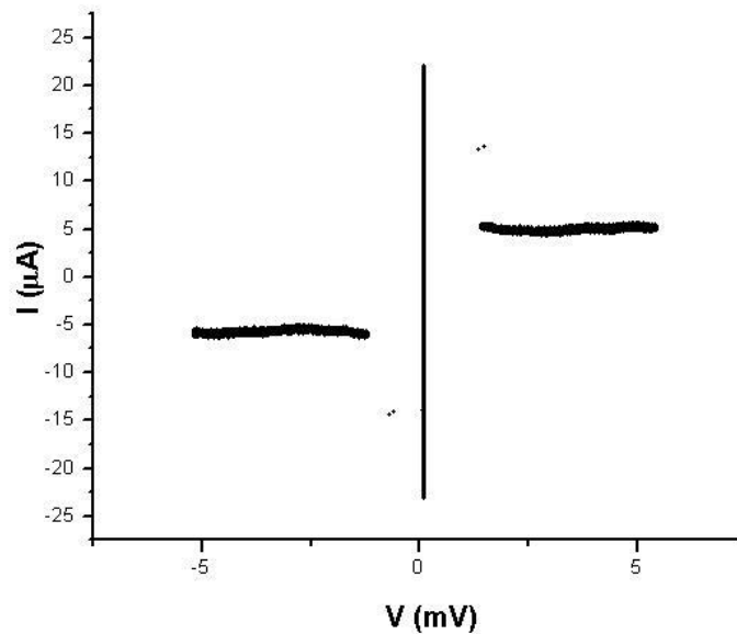
Fig. 21: Caratteristica IV a 4.2K di un hotspot plateau di un SSPD realizzato con un film di NbN su MgO spesso 7nm. I_c= 24.8\mu A , I_{hs}=5.9\mu A .
