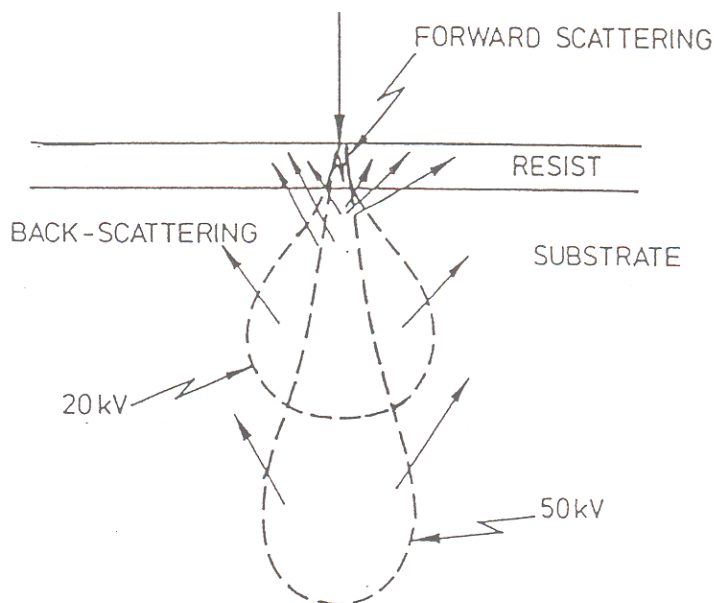
Fig. 69: Meccanismo fisico dell'effetto di prossimità
