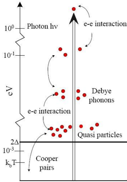
Fig. 3: Schema del processo di termalizzazione.
