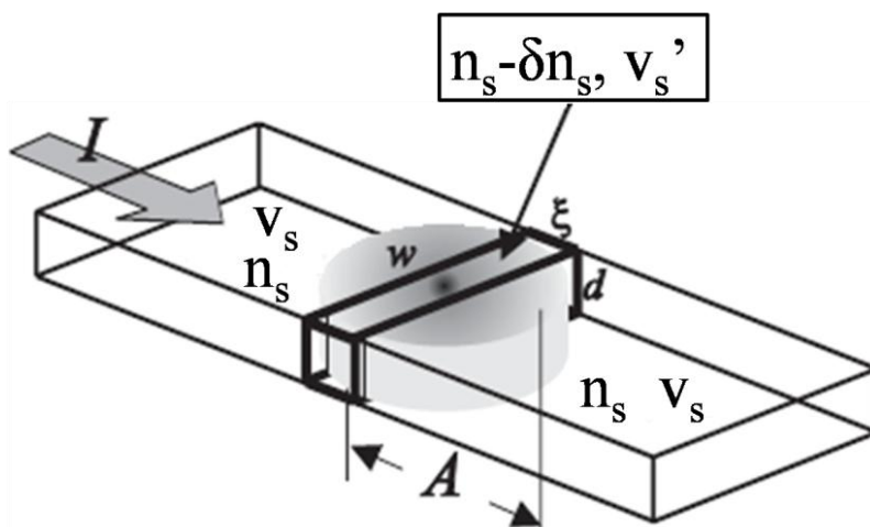
Fig. 5: Schema del nanofili superconduttore polarizzato con una corrente I . Con le linee in grassetto è indicato il volume minimo all'interno del quale una riduzione delle coppie di Cooper causa una cambiamento nella loro velocità media. Il cilindro grigio raffigura la nube di quasiparticelle di dimensione A .
