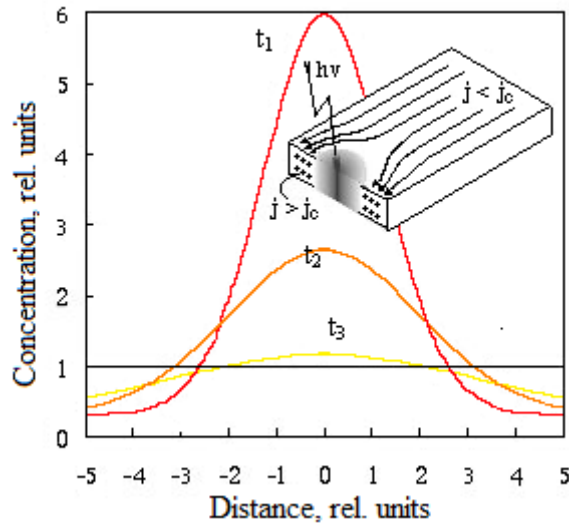
Fig. 4: Concentrazione delle quasiparticelle all'interno della sezione del filo ad istanti successivi all'assorbimento del fotone; nel riquadro è rappresentato lo schema del processo.
