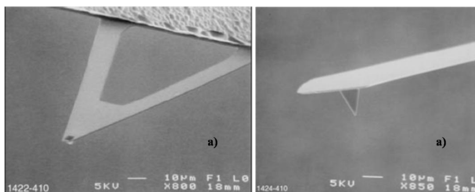
Fig. 41: Immagini SEM a) di una sonda in nitruro di silicio, b) in silicio cristallino
