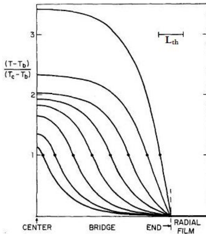
Fig. 19: Distribuzione delle temperature per diversi diametri dell' hotspot in approssimazione di L_{th} \ll 1 , assumendo che la temperatura agli estremi del film sia T=T_b . la distribuzione della restante metà del film è simmetricamente uguale. I punti riportati indicano la posizione dell'interfaccia normale superconduttore dove T=T_c .
