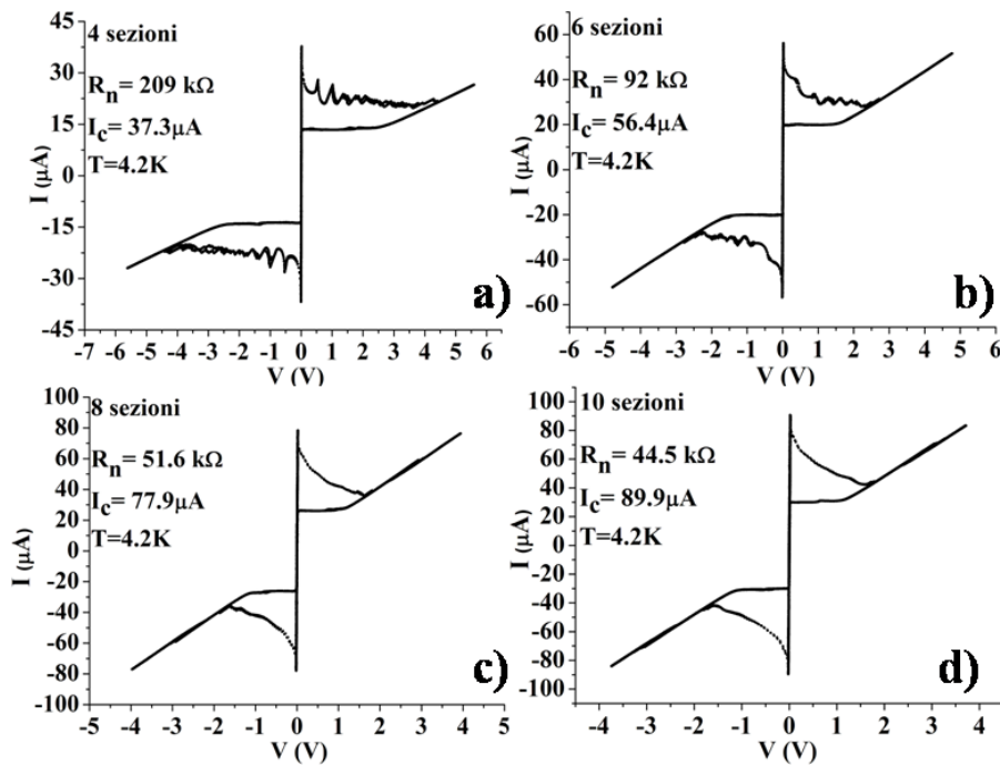
Fig. 93: Caratteristiche IV a 4.2K di diversi esempi di PND ogni sezione parallela è costituita da dei meandri in cui le dimensioni del nanofilo sono sempre le stesse w=100\text{nm} , l=10\mu\text{m} , d=5\text{nm} e f=40\% le diverse strutture differiscono tra loro per il numero di sezioni in parallelo ( N_p ) e per il numero di nanofili che costituiscono ogni elemento ( N_s ). a) PND costituito da 4 elementi in parallelo ciascuno dei quali formato dalla serie di 11 nanofili b) struttura con N_p=6 e N_s=7 , c) N_p= 8 e N_s=5 , d) N_p= 10 e N_s=5 . Come si può notare la corrente critica è all'incirca proporzionale a I_{c,\text{tot}}=N_p \times I_{c,i} , dove per esempio in figura I_{c,i} \sim 9\mu\text{A} .
