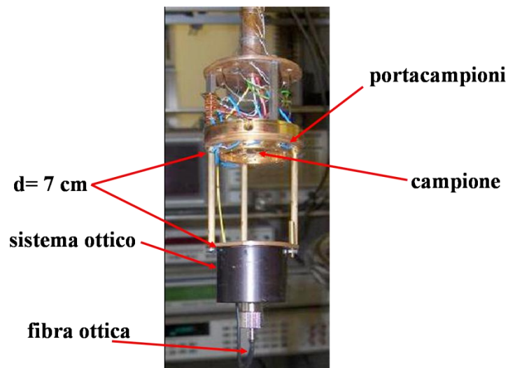
Fig. 51: Schema della parte finale dell'inserto criogenico (testa) utilizzato per la caratterizzazione ottica a 4.2K. Con le frecce rosse sono indicate le parti più significative del terminale.
