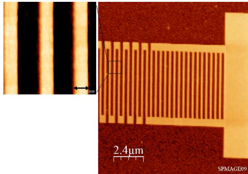
Fig. 73: Immagine al microscopio a forza atomica AFM di un SSPD realizzato su di un film di NbN su GaAs. Il fattore di riempimento del meandro è pari al 40% e la larghezza del nanofilo è pari a 100nm
