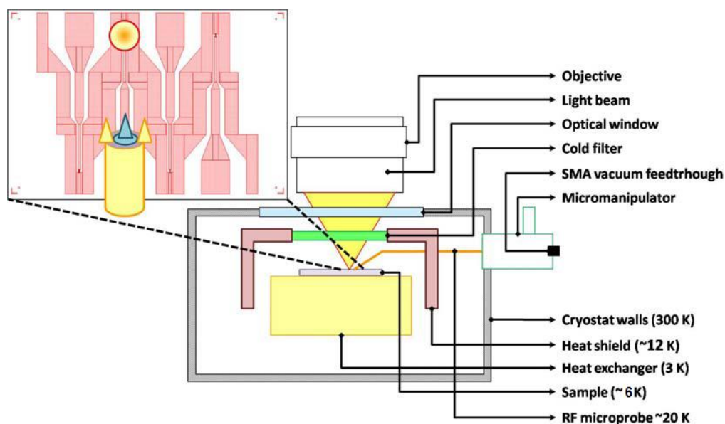
Fig. 53: Schema della probe station criogenica.
