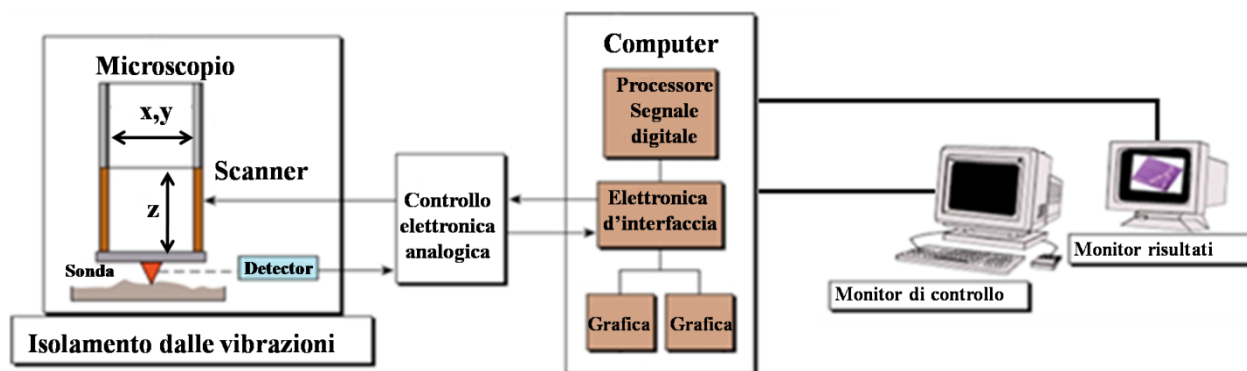
Fig. 38: Componenti di base nella SPM.
