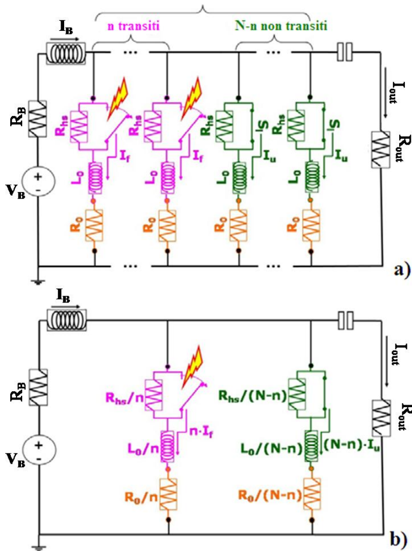
Fig. 22: a) Circuito equivalente di un N-PND con resistenze serie. Le n sezioni transite in seguito all'assorbimento di un fotone sono rappresentate in rosa tutte attraversate dalla stessa corrente I_f , mentre quelle che si trovano ancora allo stato superconduttivo sono in verde tutte con la stessa corrente I_u . I_{out} invece è la corrente che scorre attraverso la resistenza d'ingresso degli amplificatori. b) circuito semplificato dello stesso N-PND, dove i due insiemi di sezioni transite e non sono stati sostituiti dai rispettivi circuiti equivalenti di Thévenin.
