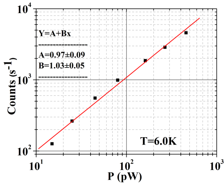
Fig. 84: Andamento dei conteggi del rivelatore in funzione della potenza del laser incidente, le misure mostrate sono state effettuate a 6K. Nell'inserto è riportato il risultato del fit lineare eseguito sui dati mostrati
