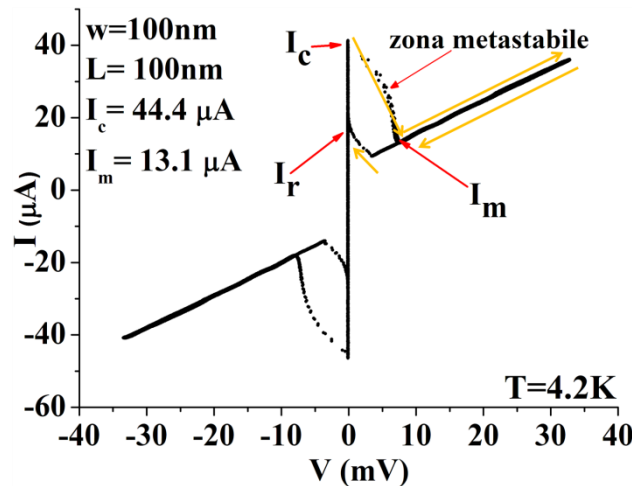
Fig. 89: Caratteristica IV a 4.2K di un SPC costituito da una struttura quadrata di dimensioni 100 \times 100 \text{nm}^2 e spessa 6nm. Seguendo le frecce gialle è possibile seguire lo sviluppo della transizione del dispositivo.
