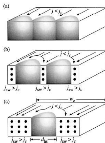
Fig.12: Schema della dinamica di formazione della zona resistiva; a) flusso di fotoni incidenti molto alto; b) regime di due fotoni per impulso che porta alla formazione di due hotspot all'interno del filo; c) regime di un singolo fotone per impulso [40].
