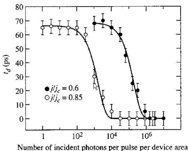
Fig. 13: Dati sperimentali ricavati per t_d da Zhang et al. in funzione del numero di fotoni incidenti per impulso laser e per unità di area del dispositivo. Le linee solide servono solo per facilitare la lettura dei dati [40].
