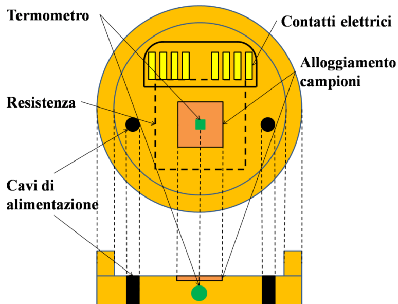
Fig. 47: Schema illustrativo del porta campioni utilizzato per la caratterizzazione elettrica dei film in elio liquido.
