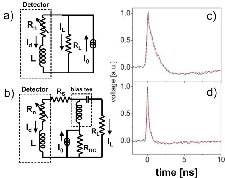
Fig. 17: a) Modello elettrico del funzionamento del dispositivo, un fotone genera un hotspot con resistenza in serie con l'induttanza cinetica del nanofilo L ; b) schema del circuito sperimentale utilizzato in [61], in cui compaiono anche la resistenza serie R_s , il bias-tee e l'impedenza del generatore di corrente; c) e d) Impulsi di risposta del rivelatore mediati per R_s = 0.250 \Omega ( L = 50 \text{ nH} ).
