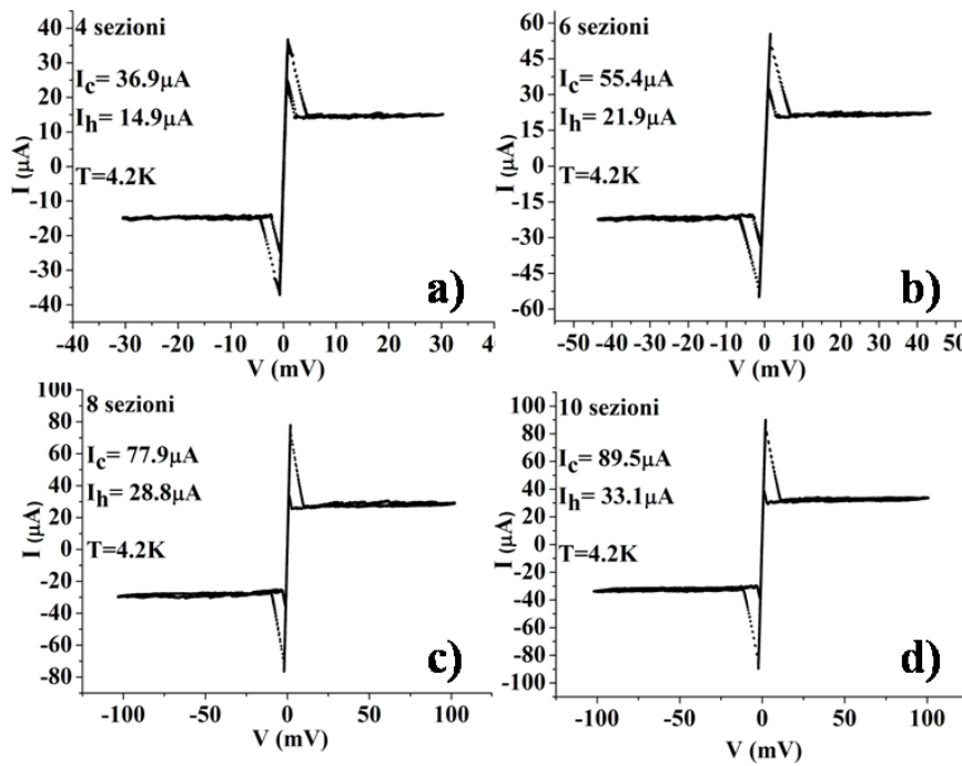
Fig. 94: Caratteristiche IV di hotspot a 4.2K di diversi esempi di PND ogni sezione parallela è costituita da dei meandri in cui le dimensioni del nanofilo sono sempre le stesse w=100nm , l=10\mu m , d=5nm e f=40\% . Le diverse strutture differiscono tra loro per il numero di sezioni in parallelo ( N_p ) e per il numero di nanofili che costituiscono ogni elemento ( N_s ). a) PND costituito da N_p=4 elementi in parallelo ciascuno dei quali formato dalla serie di N_s=11 nanofili b) struttura con N_p=6 e N_s=7 , c) N_p= 8 e N_s=5 , d) N_p= 10 e N_s=5 . Come si può notare anche la corrente di hotspot I_h , oltre alla corrente critica, è all'incirca proporzionale a N_p , dove per esempio in figura I_{h,i} \sim 3.5\mu A .
