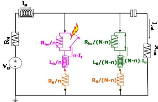
Fig. 97: Circuito equivalente di un N-PND con resistenze serie utilizzato per simulare il funzionamento del rivelatore.
