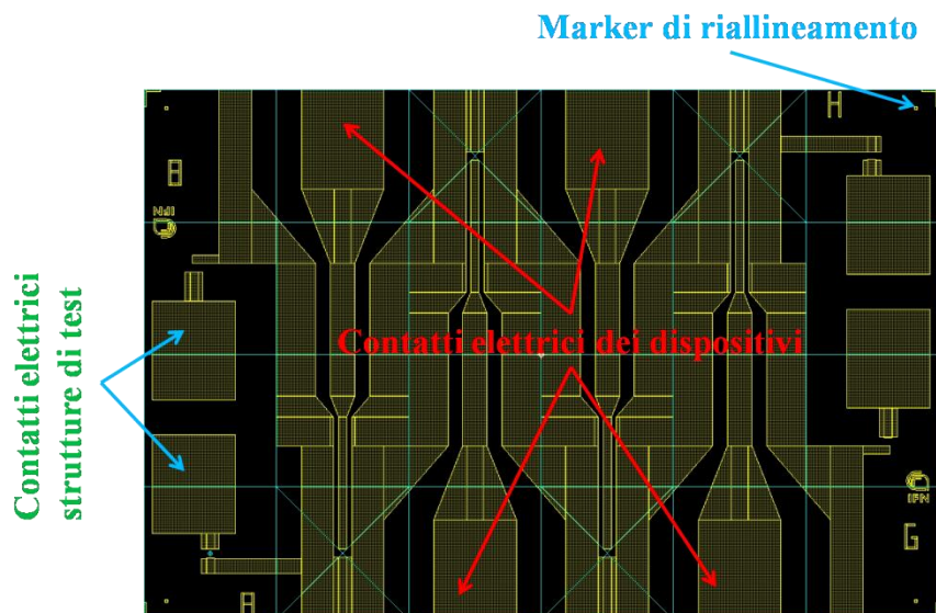
Fig. 66: Disegno dei contatti elettrici adattati a 50Ω utilizzati per la caratterizzazione di tutti i nostri dispositivi; in figura inoltre sono indicati con le frecce rosse sia i marker di riallineamento negli step successivi, sia i contatti elettrici dei quattro dispositivi inseriti in ogni chip.
