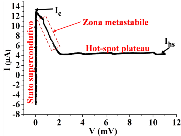
Fig. 79: Caratteristica IV di un hotspot plateau misurata a 4.2K. In figura sono indicate le tre zone: superconduttiva, metastabile e la regione dell' hotspot plateau .
