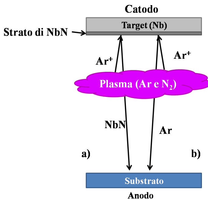
Fig. 55: Schema dei due processi antagonisti che avvengono durante il processo di sputtering. a) uno ione argon viene accelerato verso il catodo e interagendo con il target rimuove una particella di NbN, b) uno ione argon accelerato verso il target ne riemerge come un atomo neutro. I due processi sono rappresentati separatamente per semplicità, in realtà l'arrivo di uno ione provoca il distacco di un atomo di NbN e la riflessione di un atomo di Ar.
