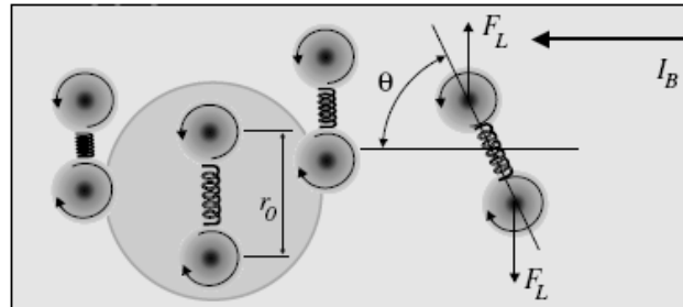
Fig. 11: Schema illustrativo del modello dei VAP per un evento di dark count in un filo superconduttore. Il nanofilo è polarizzato con una corrente I_B , la forza di Lorentz agisce su entrambi i vortici di ogni VAP portando ad un orientamento preferenziale della coppia. Il cerchio rappresenta una zona in cui è presente una fluttuazione termica che può causare la rottura del legame tra i vortici.
