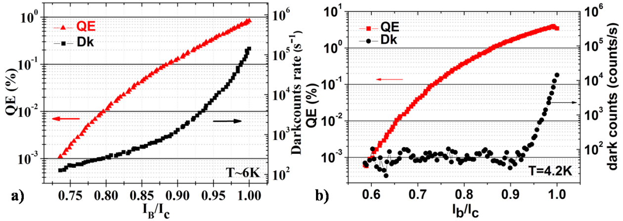
Fig. 88: a) Misura dell'efficienza quantica a 6K di un SSPD costituito da un nanofilo largo 100nm spesso 5nm e disposto a meandro con un fattore di riempimento del 40%, la lunghezza d'onda della radiazione incidente è pari a \lambda = 1.3 \mu m ; b) misura dell'efficienza quantica dello stesso dispositivo a 4.2K e \lambda = 780nm .
