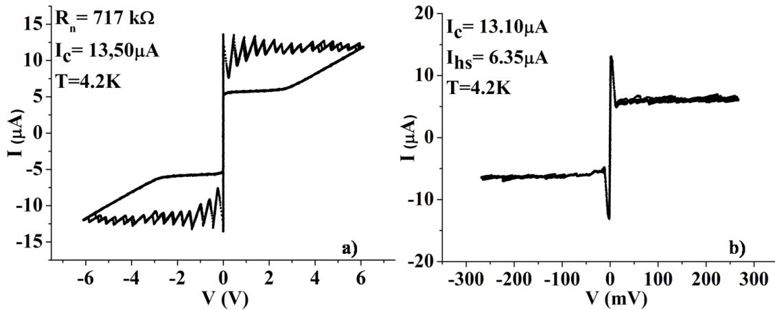
Fig. 81: a) caratteristica IV ottenute a 4.2K con un meandro costituito da un nanofilo di NbN su GaAs largo 100nm, lungo 105μm e spesso 5nm; b) caratteristica IV del hotspot plateau ottenuta con lo stesso dispositivo sempre a 4.2K
