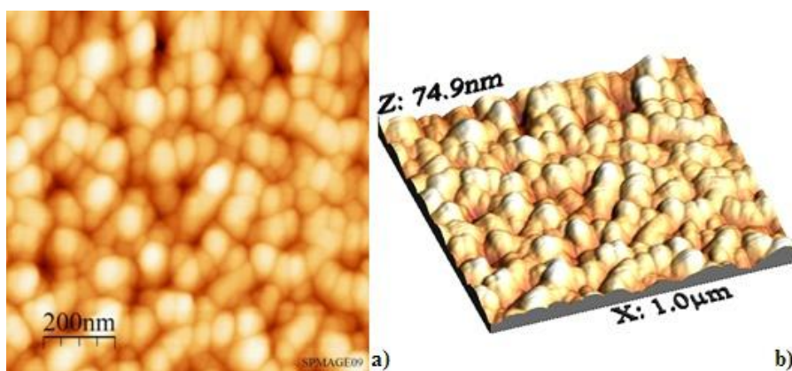
Fig. 60: a) Immagine AFM 2D della superficie di un film di NbN depositato su GaAs mantenendo il substrato ad una temperatura T_s=400^\circ\text{C} , l'area di scansione è di 1\mu\text{m}^2 , b) la stessa immagine in 3D.
