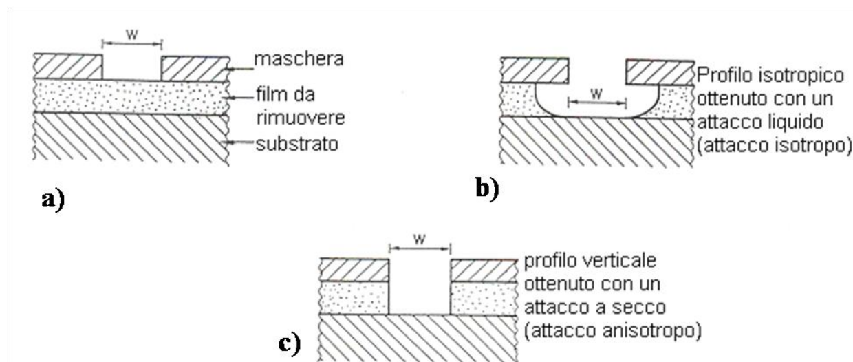
Fig. 34: a) Sezione trasversale di un campione prima di effettuare l'attacco; b) Sezione trasversale di un campione sottoposta ad etching liquido; b)risultato ottenibile con un attacco a secco.
