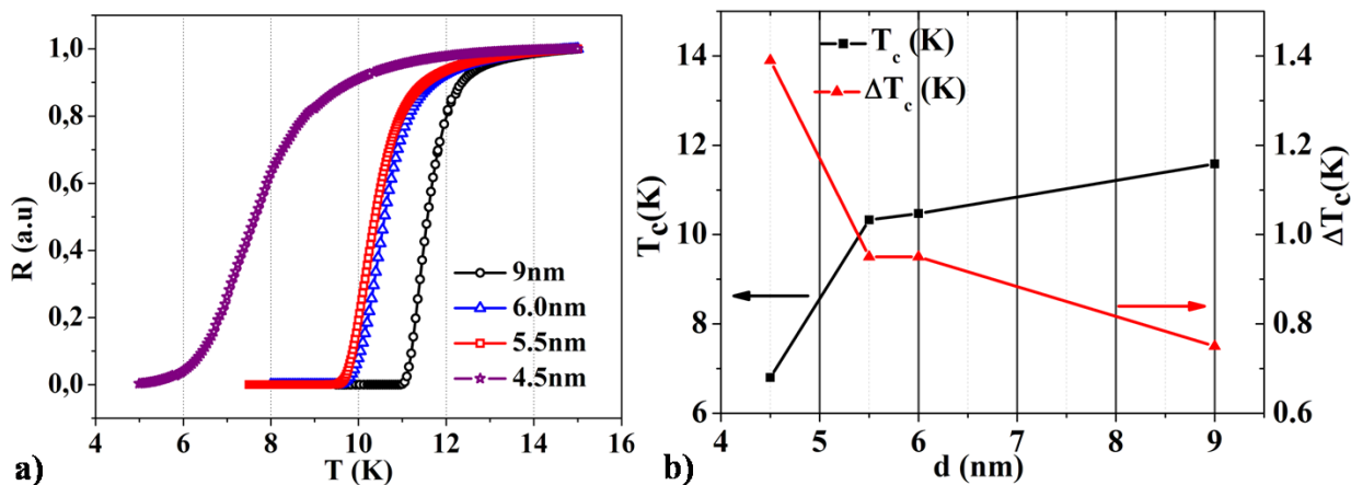
Fig. 58: a) Resistenza dei film di NbN su GaAs di vari spessori in funzione della temperatura; b) andamento della temperatura critica e della larghezza di transizione in funzione dello spessore.
