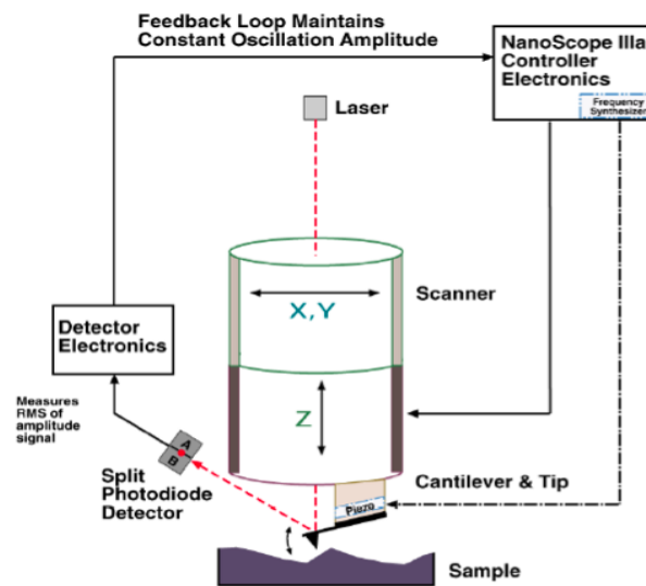
Fig. 39: Schema di AFM in Tapping Mode
