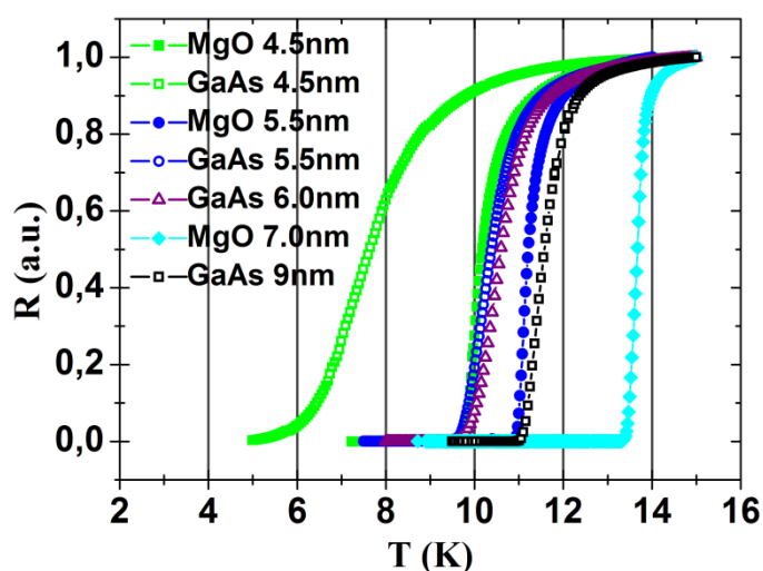
Fig. 59: Confronto tra film di diversi spessori depositi su MgO (simboli pieni) e film depositi su GaAs (simboli aperti); colori uguali corrispondono a spessori nominali uguali.
