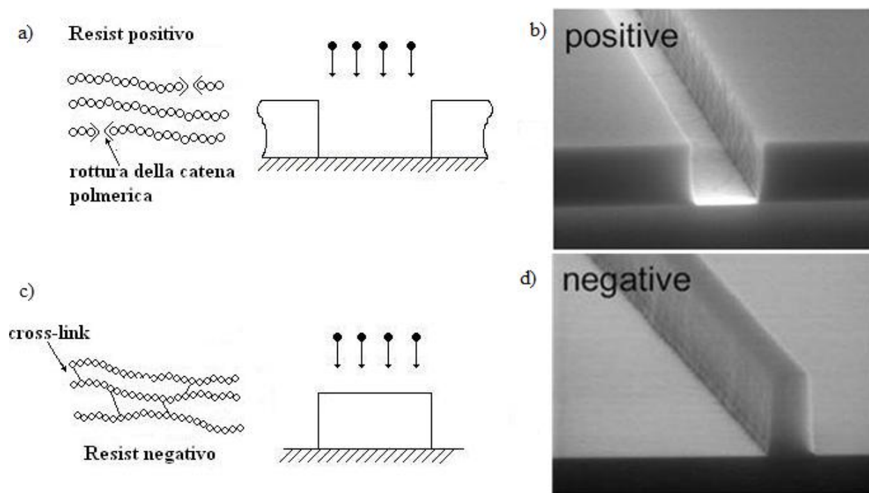
Fig. 25: a) Descrizione schematica del comportamento di un resist positivo, b) immagine SEM relativa ad un resist positivo, c) descrizione schematica del comportamento di un resist negativo con corrispondente immagine SEM d).
