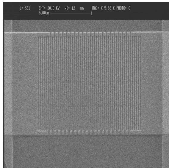
Fig. 1: Immagine al microscopio a scansione elettronica (SEM) di un SSPD costituito da un nanofilo, largo 100nm spesso 4.5nm, disposto a meandro, la spaziatura tra due porzioni adiacenti del nanofilo è pari a 150nm, ognuna è lunga 10 \mu\text{m} e il loro numero totale è 21. L'area totale è pari a 100 \mu\text{m}^2 .
