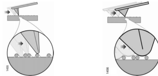
Fig. 42: Esempio di scansione con punte di forma diversa
