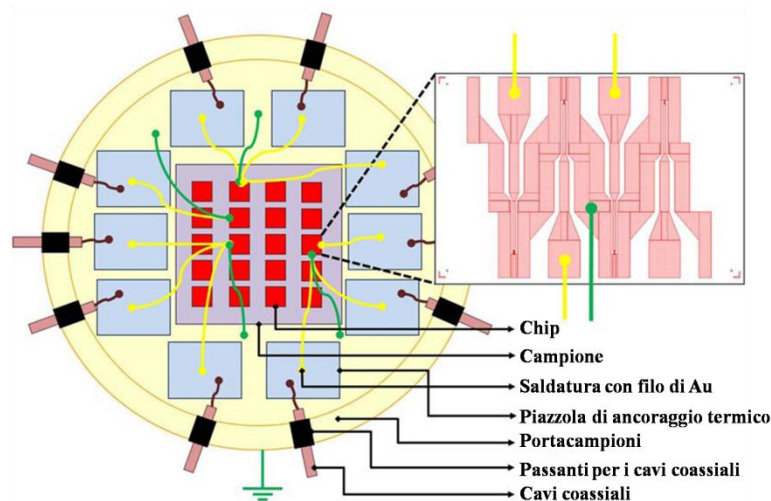
Fig. 50: Immagine del porta campioni utilizzato per le misure ottiche in elio liquido a 4.2K. In giallo sono evidenziate le saldature di Au utilizzate per la connessione dei contatti elettrici dei dispositivi, mentre in verde sono indicate le connessioni a massa dei dispositivi
