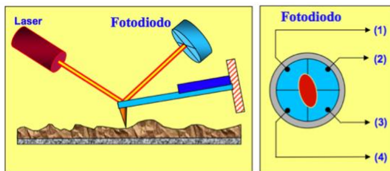
Fig. 40: Schema del sistema di rilevamento delle flessioni della leva con metodo ottico.
