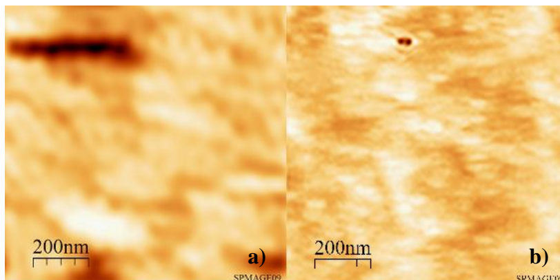
Fig. 63: Immagini AFM delle superfici dei campioni di GaAs utilizzati per determinare il valore massimo di T_s per un tempo di riscaldamento breve, a) mantenendo il substrato a 300°C per 7h e 30' e a 400°C per soli 30'; b) mantenendo il substrato a 300°C per 7h e 30' e a 350°C per soli 30'
