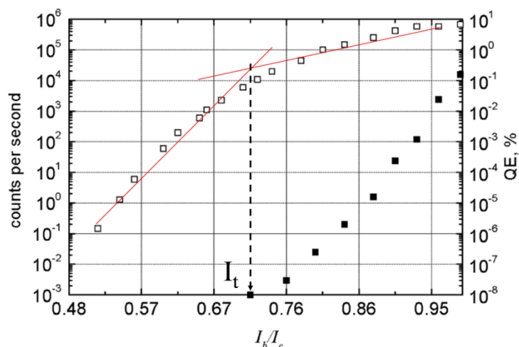
Fig. 6: Conteggi al secondo di un SSPD (simboli vuoti) e dei dark count (simboli pieni) in funzione della corrente di polarizzazione I_b normalizzata rispetto alla corrente critica I_c . Lo spessore del film di NbN è di 3.5nm. L'asse di destra rappresenta la corrispondente efficienza quantica. Le linee rosse sono state aggiunte per rendere più facile la visualizzazione del cambio di pendenza nell'andamento della QE al disotto di I_t indicata dalla linea tratteggiata.
